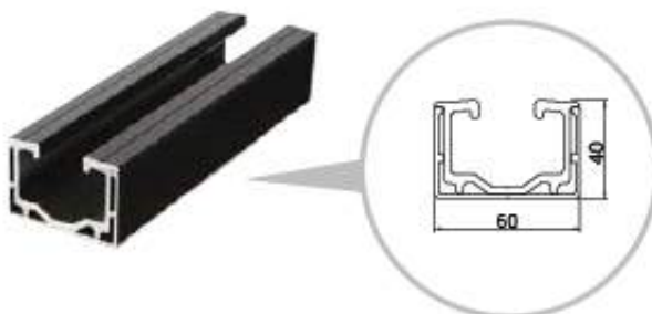
일반형 하부레일, 프로파일 이미지 및 상세도
