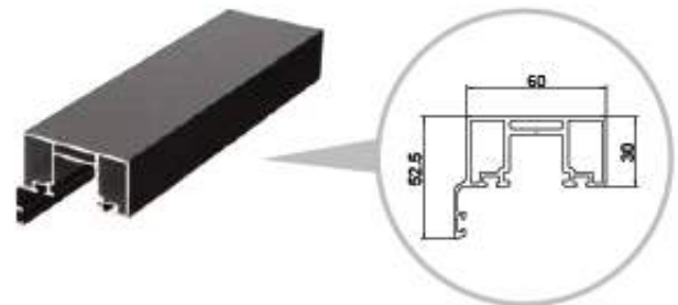
창문형 하부레일, 프로파일 이미지 및 상세도
