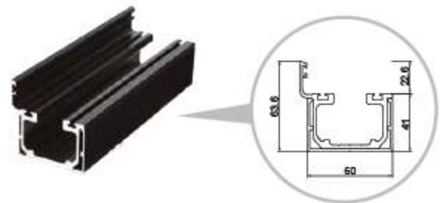
창문형 하부레일, 프로파일 이미지 및 상세도
